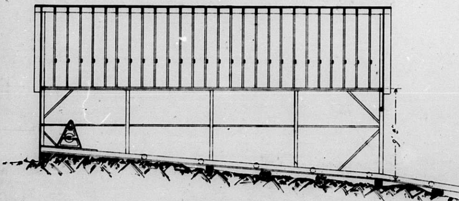
LONGITUDINAL SECTION.
