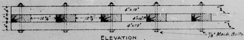
ELEVATION
