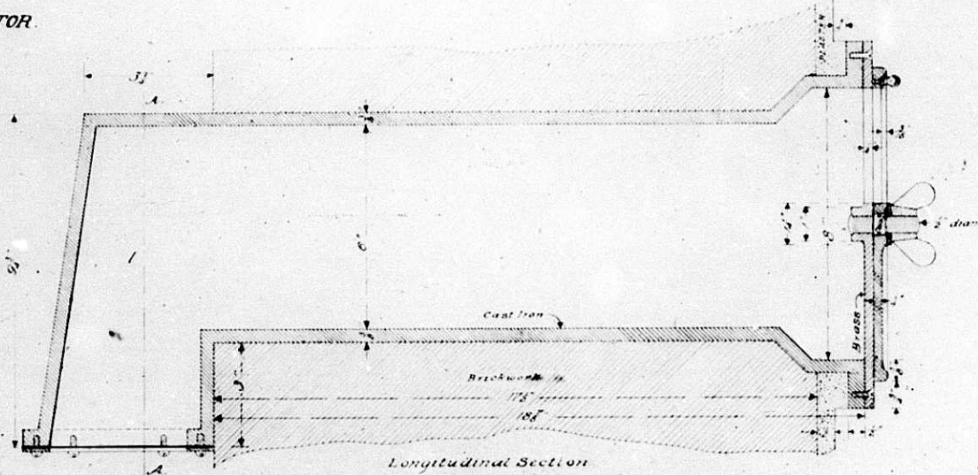
Longitudinal Section
